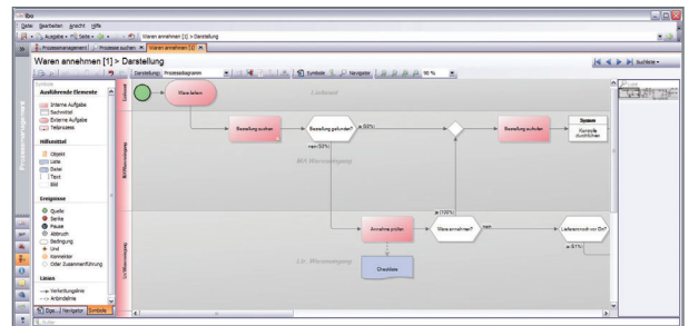
Prozessdiagramm
