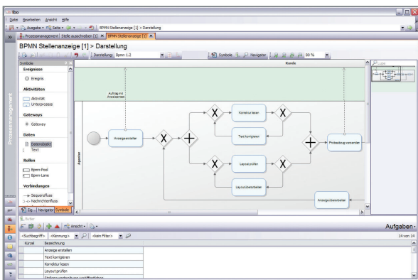
Modellierungsstandard BPMN
